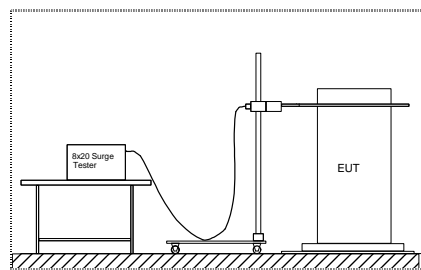
EUT setup
